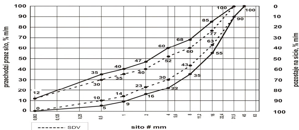
Rys. 2. Uziarnienie mieszanki niezwiązanej 0/31,5 dla podbudowy pomocniczej
