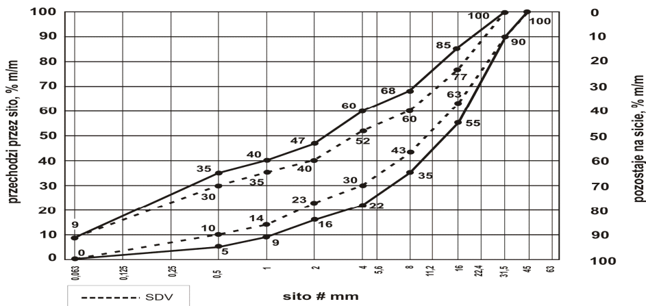
Rys. 3. Uziarnienie mieszanki niezwiązanej 0/31,5 dla podbudowy zasadniczej
