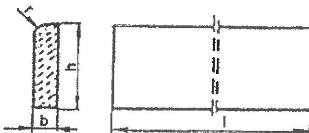
Rysunek 1. Kształt betonowego obrzeża chodnikowego
