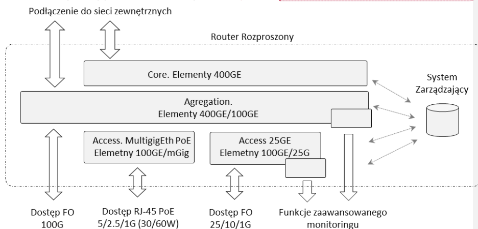
Rysunek 1 Schemat funkcjonalny routera rozproszonego
