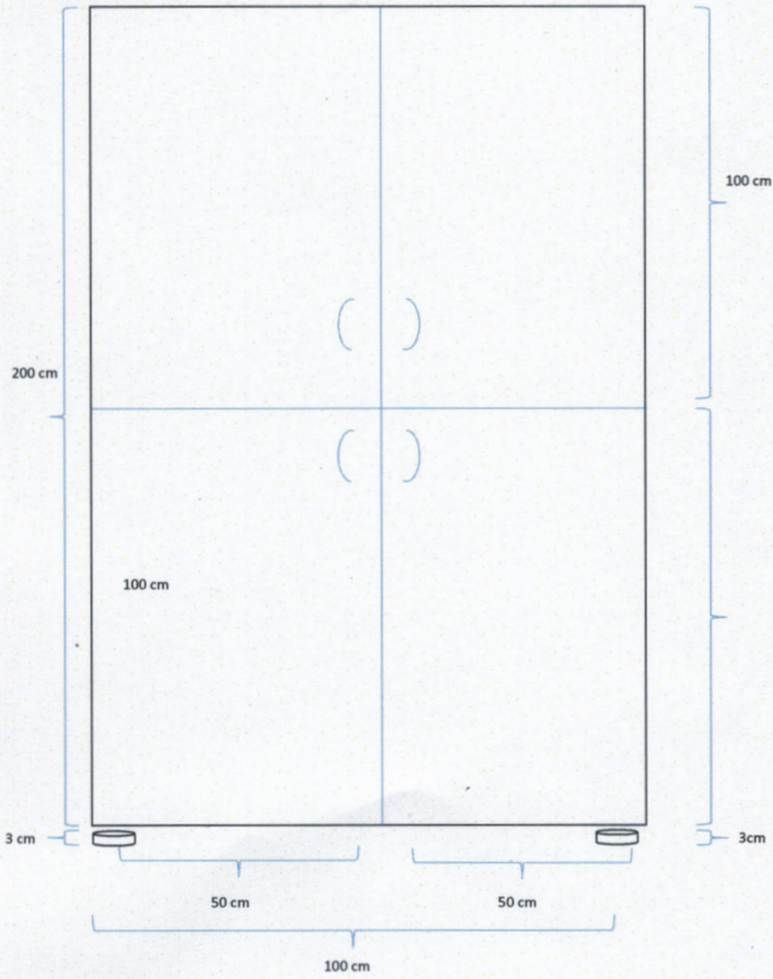
Szafa na dokumenty zamknięta – widok z przodu
