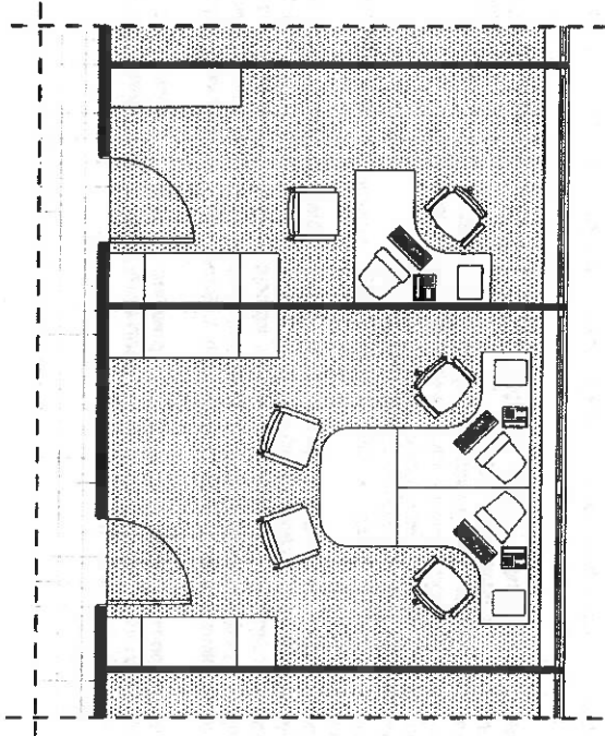
Rys. nr 6. Przykładowy układ funkcjonalny pomieszczeń biurowych 2 osobowych i 1 osobowych z wyposażeniem.
