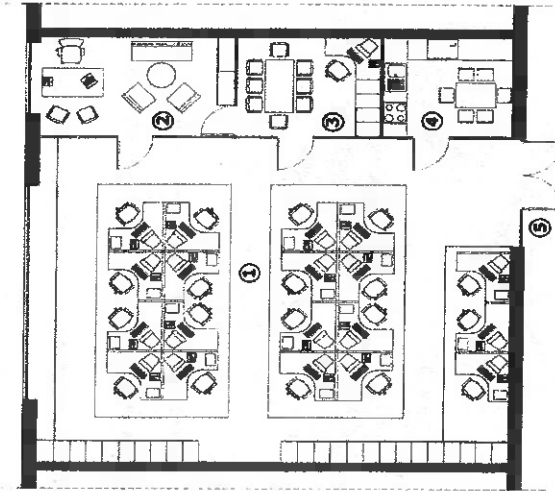
Rys. nr 4. Przykładowy schemat pomieszczenia pracy zespołowej stałej: 1. Pomieszczenie ogólne pracy; 2. pomieszczenie biurowe przelozone; 3. mała sala odpraw; 4. pokój socjalny; 5. komunikacja ogólna obiektu.
