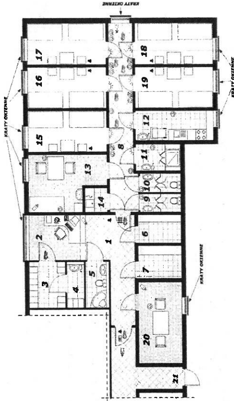
Rys. nr 10. Przykładowy układ funkcjonalny (PdOZ):
