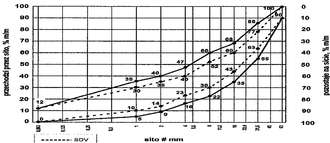
Rysunek 2. Mieszanka kruszyw 0/31,5 do górnej warstwy nawierzchni
