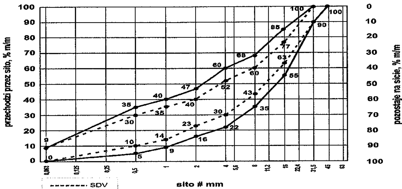
Rysunek 2. Mieszanka kruszyw 0/31,5 do górnej warstwy nawierzchni
