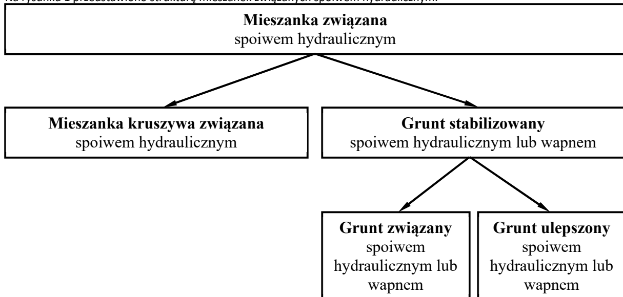
Rysunek 1 Struktura mieszanek związanych spoiwem hydraulicznym
