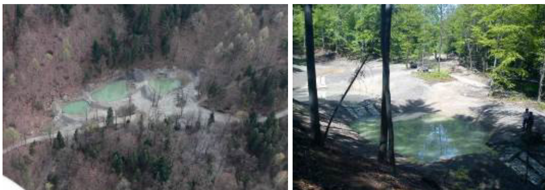
Odbudowa 3 zbiorników w układzie kaskadowym w N-ctwie Bielsko
