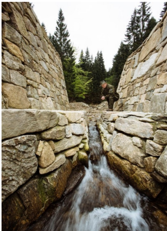
V-kształtny przelew wody ze zbiornika przeciwpowodziowego umożliwiający przejście rumowiska i samoczynne napełnianie i opróżnianie obiektu - Nadleśnictwo Międzylesie. Źródło: Archiwum CKPŚ. (rys. z prawej strony)
