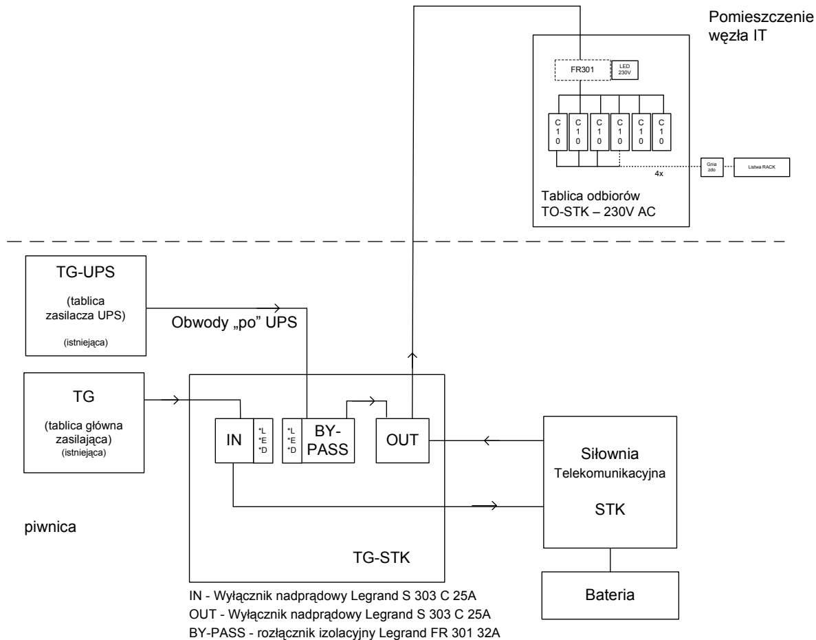
Rysunek 1 – Schemat połączeń – KPP Ropczyce
