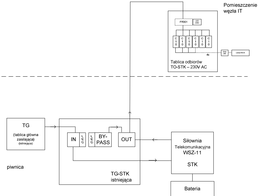
Rysunek 2 – Schemat połączeń – KPP Mielec
