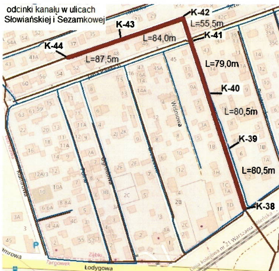
Rys.2 Lokalizacja odciniek kolektora w ul. Słowiańskiej i Sezamkowej w Ząbkach
