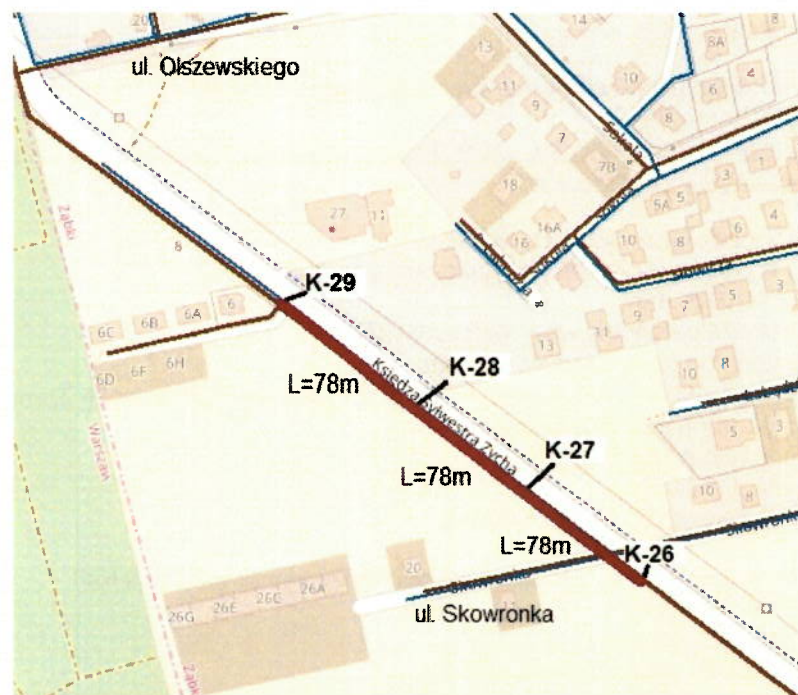
Rys.1 Lokalizacja odciniek kolektora w ul. ks. Sylwestra Zycha w Ząbkach
